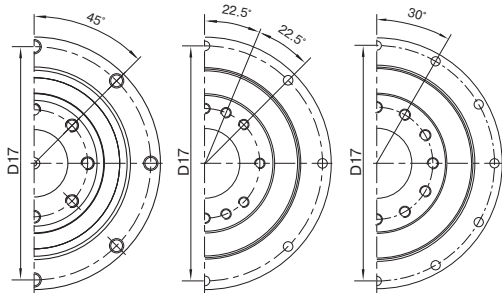
图示为带平键的 PSFN090 / 1 级 / 法兰输出轴 / 14 mm 锁紧系统 / 适配电机法兰 - 2 件式 - 圆形通用法兰 / B5 电机法兰类型
