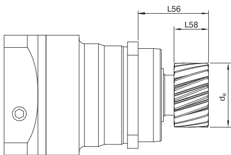
PSN/PLN 带小齿轮 (也适用于 WPLN, PLHE 和 WPLHE) PSN/PLN with pinion (also applies to WPLN, PLHE and WPLHE)
