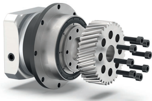
适用于 090 减速机尺寸的 PSFN090 (带有 PM1 齿轮)
