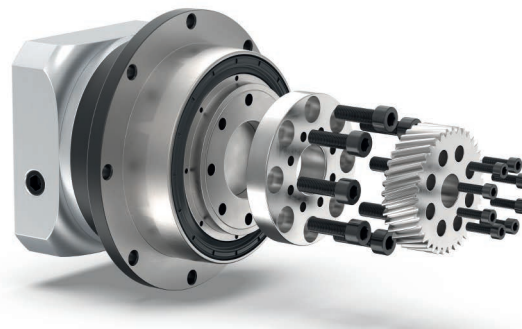
带有转接法兰的 PSFN090 (064 → 090) 与 PM1 齿轮 (适用于 064 减速机齿轮)
