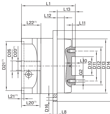
图示为带平键的 PSFN090 / 1 级 / 法兰输出轴 / 14 mm 锁紧系统 / 适配电机法兰 - 2 件式 - 圆形通用法兰 / B5 电机法兰类型
